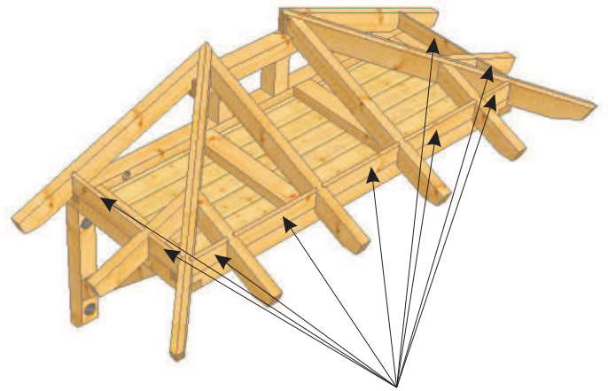
Stellbretter zwischen die Sparren
