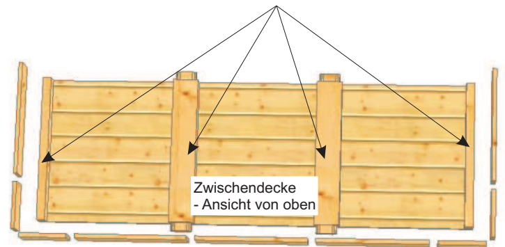
Unterkonstruktion für die Zwischendecke
